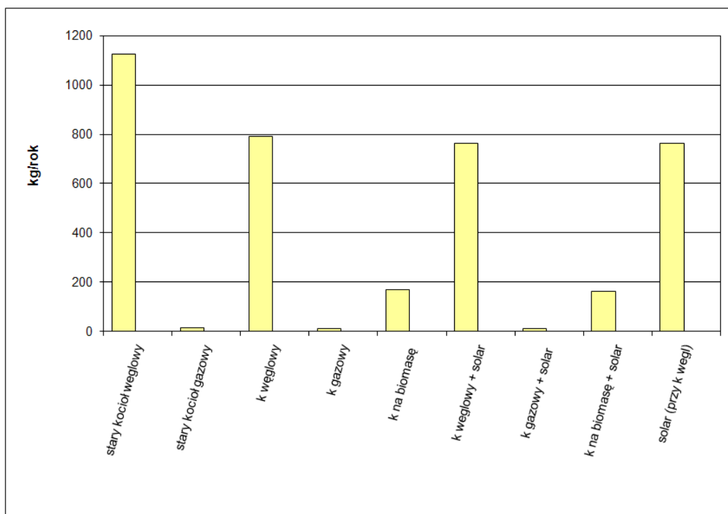
Rysunek 15. Emisja zanieczyszczeń pyłowo gazowych dla poszczególnych zakresów modernizacji
