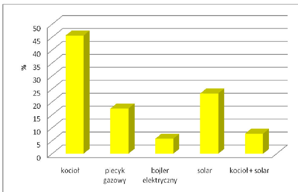
Rysunek 11. Przygotowanie ciepłej wody – po modernizacji
