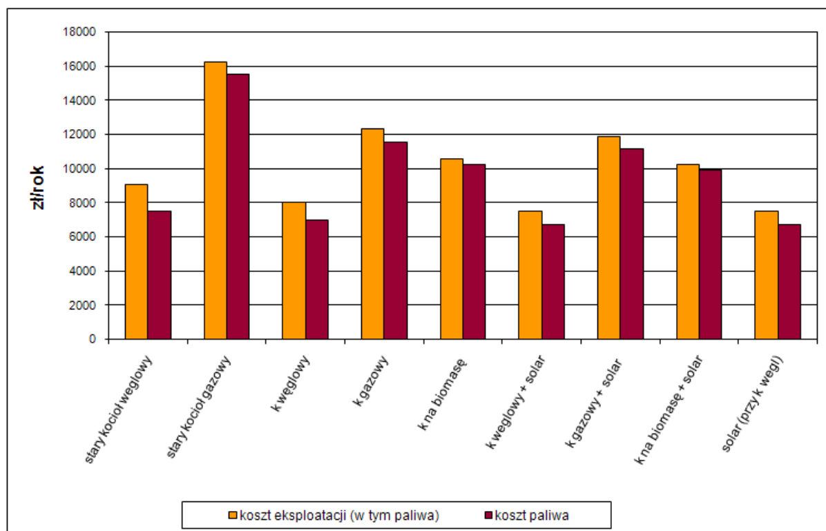
Rysunek 14. Porównanie kosztów eksploatacyjnych dla istniejącego komfortu cieplnego
