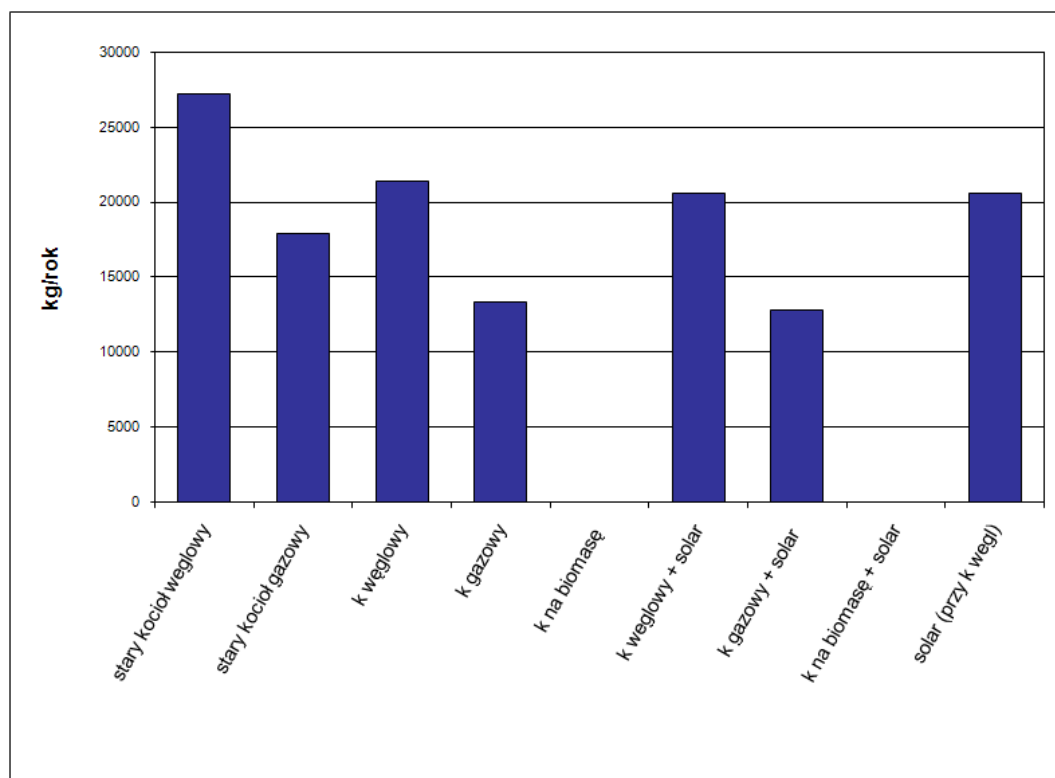
Rysunek 16. Emisja dwutlenku węgla dla poszczególnych zakresów modernizacji
