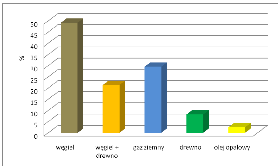
Rysunek 5. Struktura stosowanego paliwa przed planowaną modernizacją
